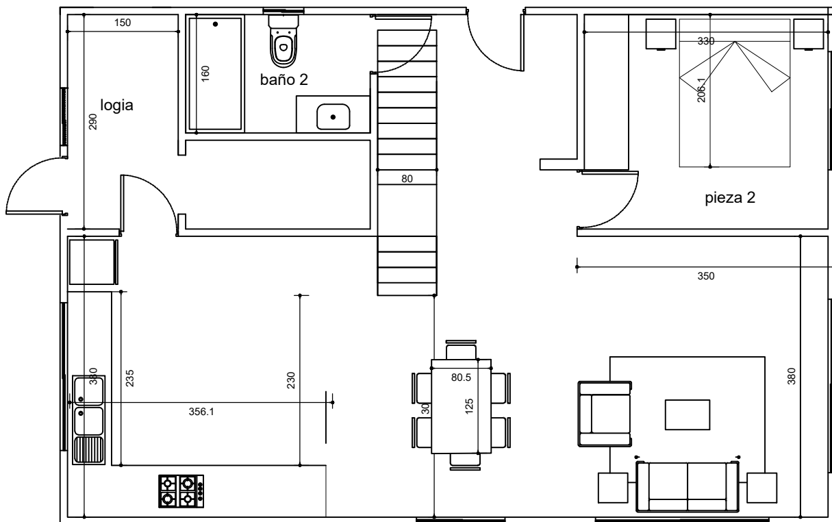
1er Piso
